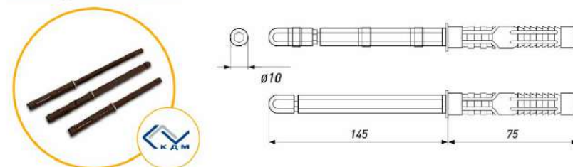
МЕНСОЛОДЕРЖАТЕЛЬ 10*145
