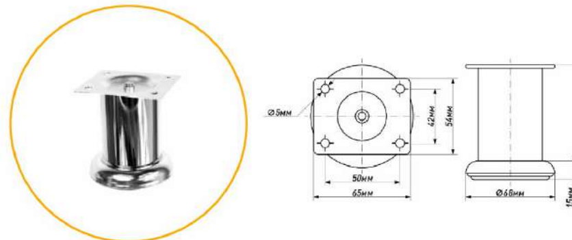
ОПОРА МЕБЕЛЬНАЯ (КРУГЛАЯ)
