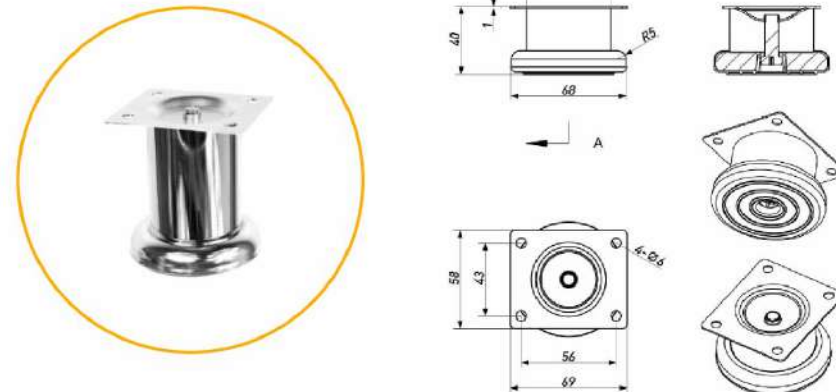
ОПОРА МЕБЕЛЬНАЯ (КРУГЛАЯ)
