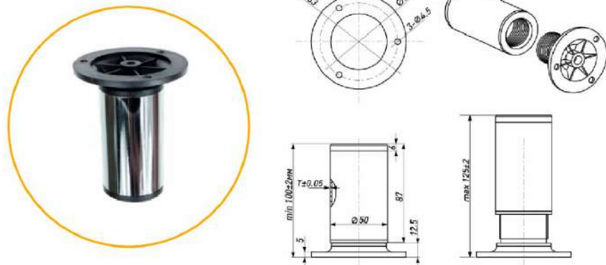
ОПОРА МЕБЕЛЬНАЯ ЦОКОЛЬНАЯ
