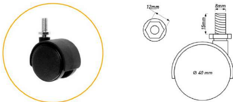
ОПОРА КОЛЁСНАЯ (НА РЕЗЬБЕ)
