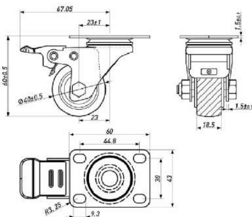
ОПОРА КОЛЁСНАЯ УСИЛЕННАЯ (С ПОВОРОТНОЙ ПЛОЩАДКОЙ, С ТОРМОЗОМ)
