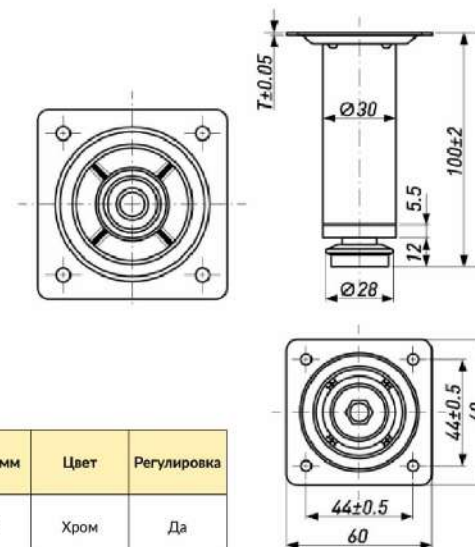
ОПОРА МЕБЕЛЬНАЯ (КРУГЛАЯ)
