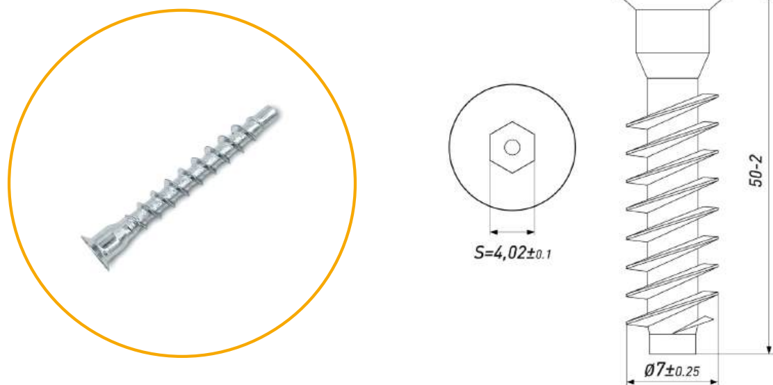
ЕВРОВИНТ 7*50
