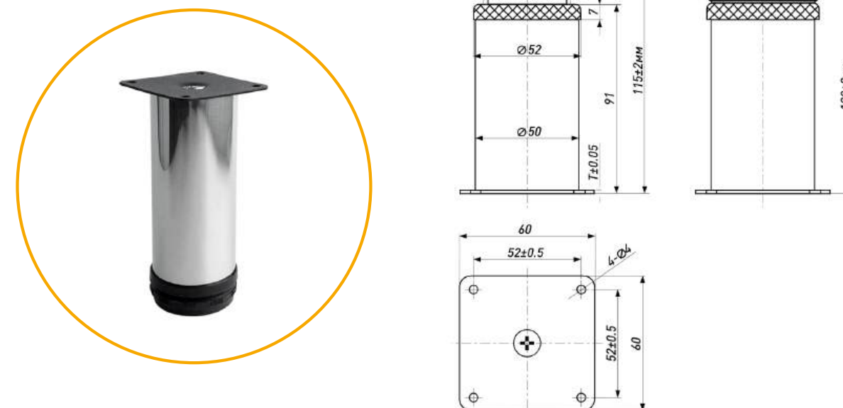
ОПОРА МЕБЕЛЬНАЯ ЦОКОЛЬНАЯ (ФЛАНЕЦ КВАДРАТ)
