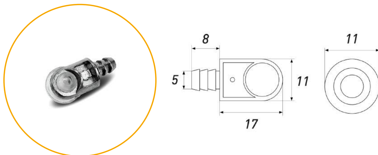
ПОЛКОДЕРЖАТЕЛЬ ДЛЯ СТЕКЛА С ПРИСОСКОЙ
