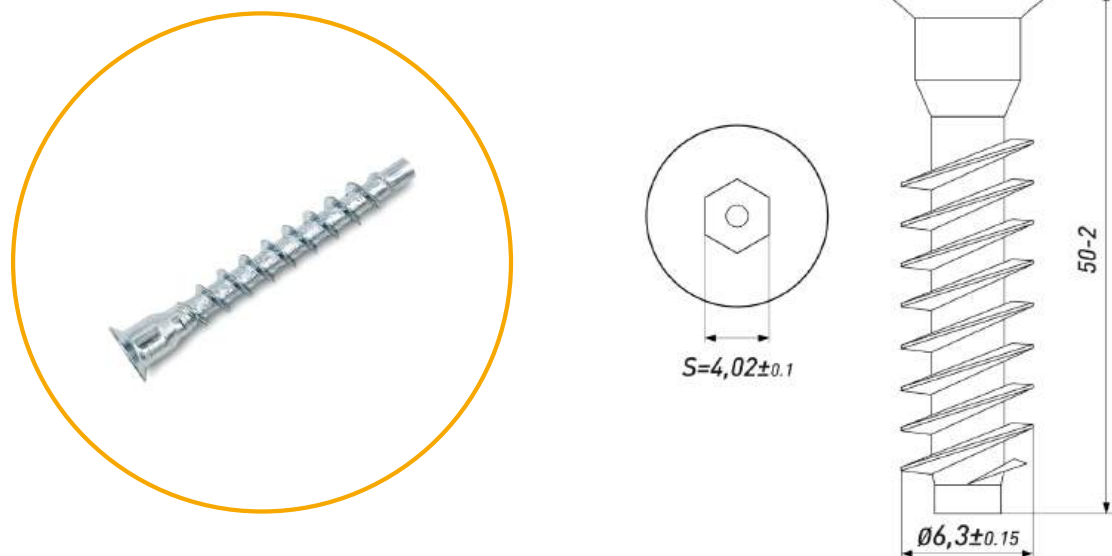
ЕВРОВИНТ 6,3*50
