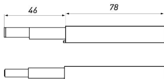
АМОРТИЗАТОР НАКЛАДНОЙ
