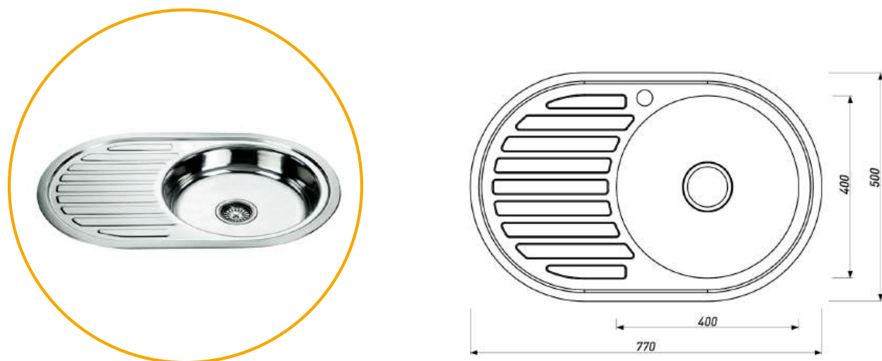
МОЙКА ОВАЛЬНАЯ (ПРАВАЯ)
