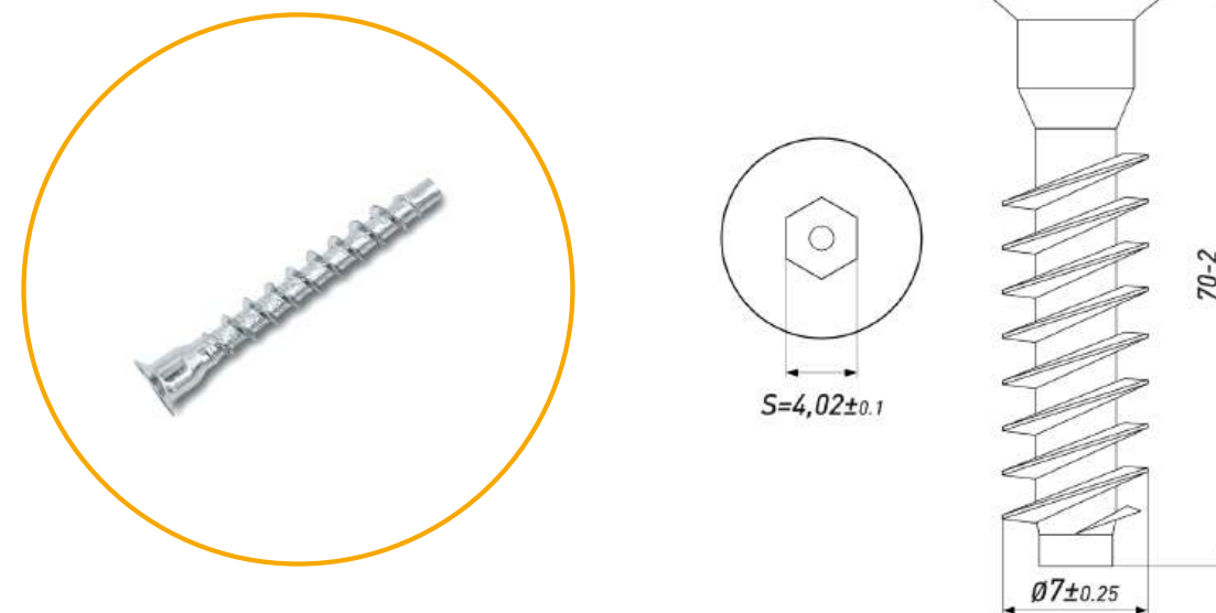
ЕВРОВИНТ 7*70
