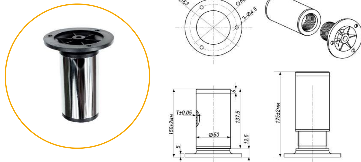
ОПОРА МЕБЕЛЬНАЯ ЦОКОЛЬНАЯ (ФЛАНЕЦ КРУГ)
