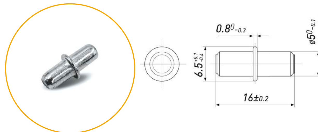
ПОЛКОДЕРЖАТЕЛЬ 5*16 МЕТАЛЛИЧЕСКАЯ ОСЬ
