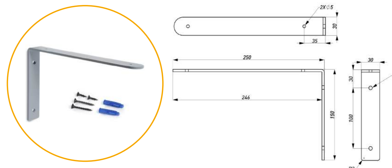
ПОЛКОДЕРЖАТЕЛЬ 1-01
