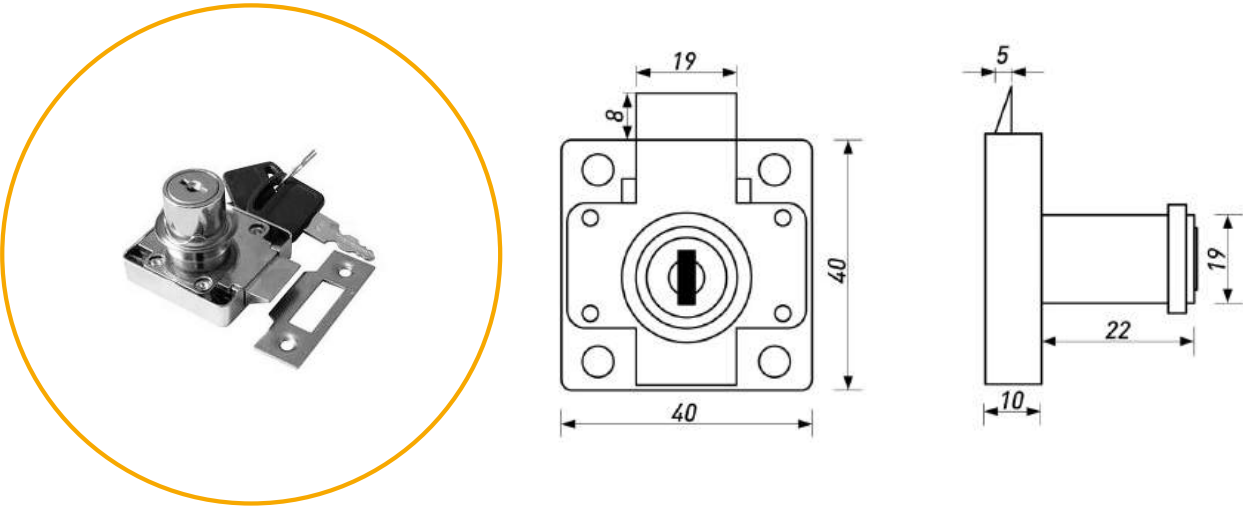
ЗАМОК МЕБЕЛЬНЫЙ № 338
