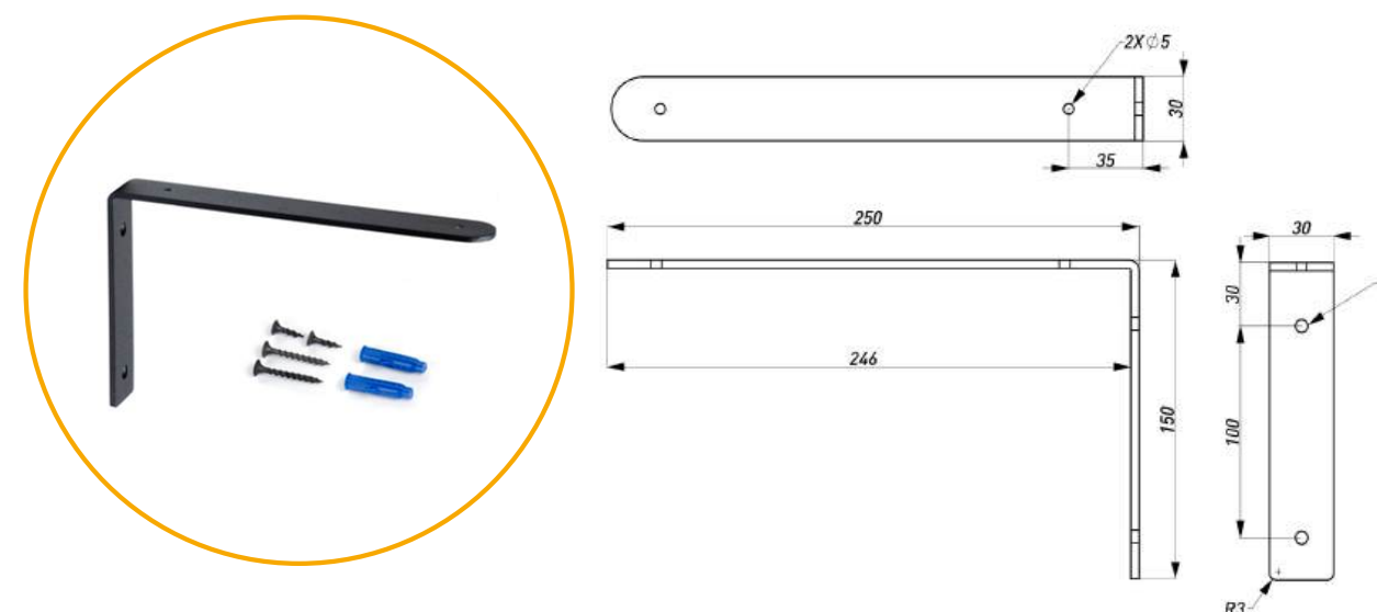
ПОЛКОДЕРЖАТЕЛЬ 1-01
