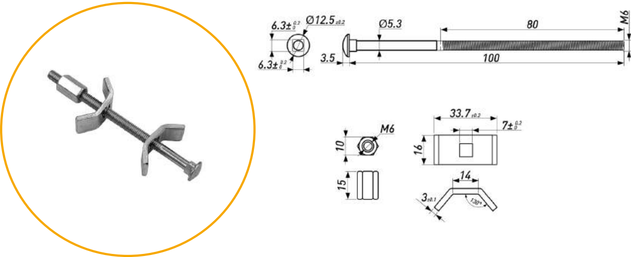
СТЯЖКА ДЛЯ СТОЛЕШНИЦЫ
