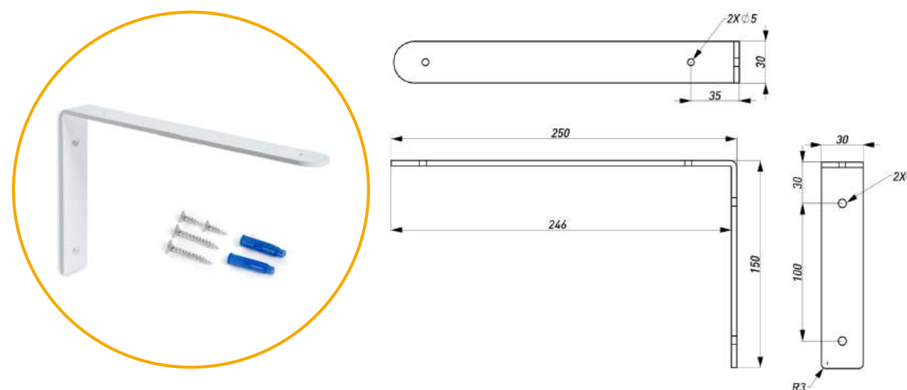
ПОЛКОДЕРЖАТЕЛЬ 1-01
