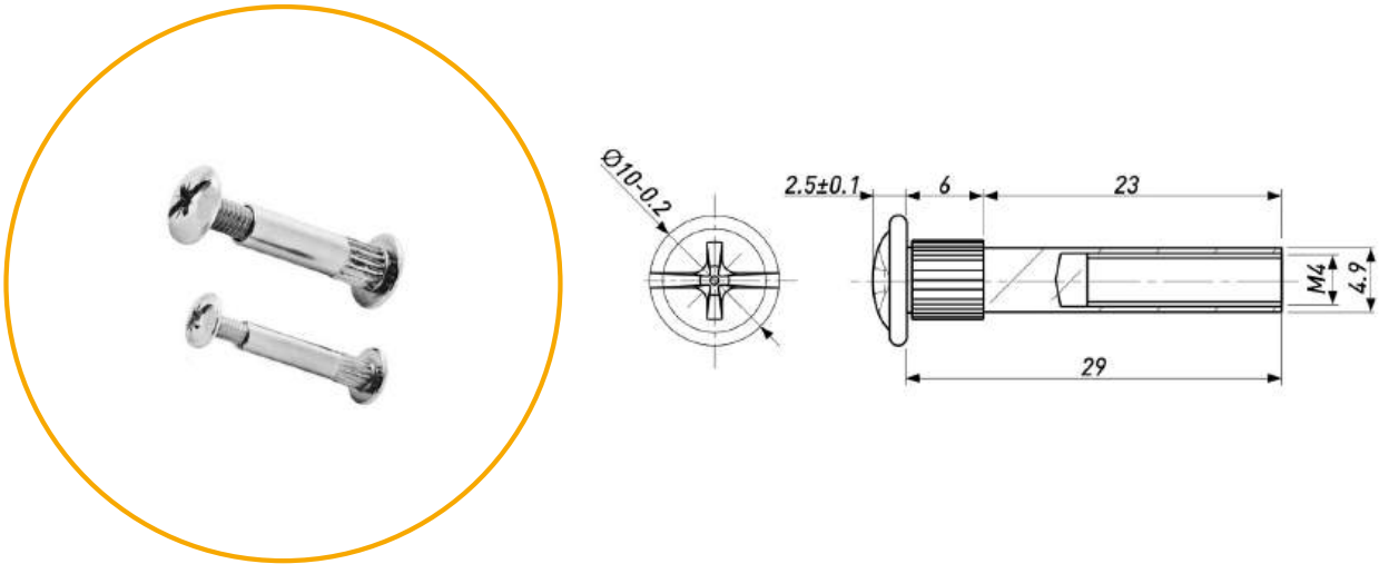
СТЯЖКА МЕЖСЕКЦИОННАЯ
