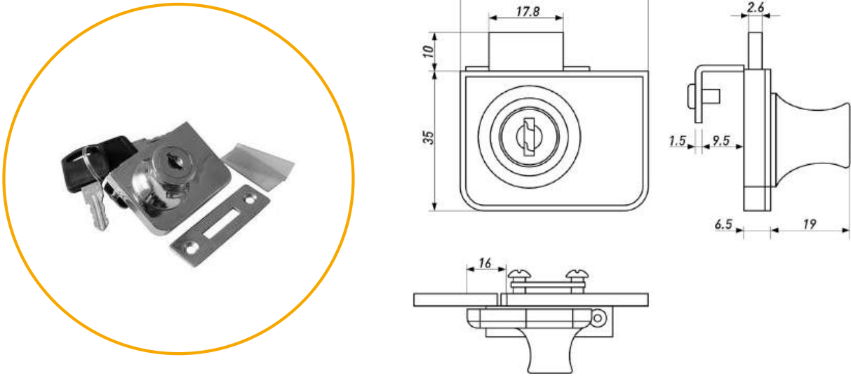
ЗАМОК МЕБЕЛЬНЫЙ № 805
