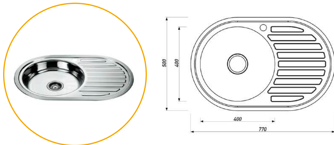
МОЙКА ОВАЛЬНАЯ (ЛЕВАЯ)
