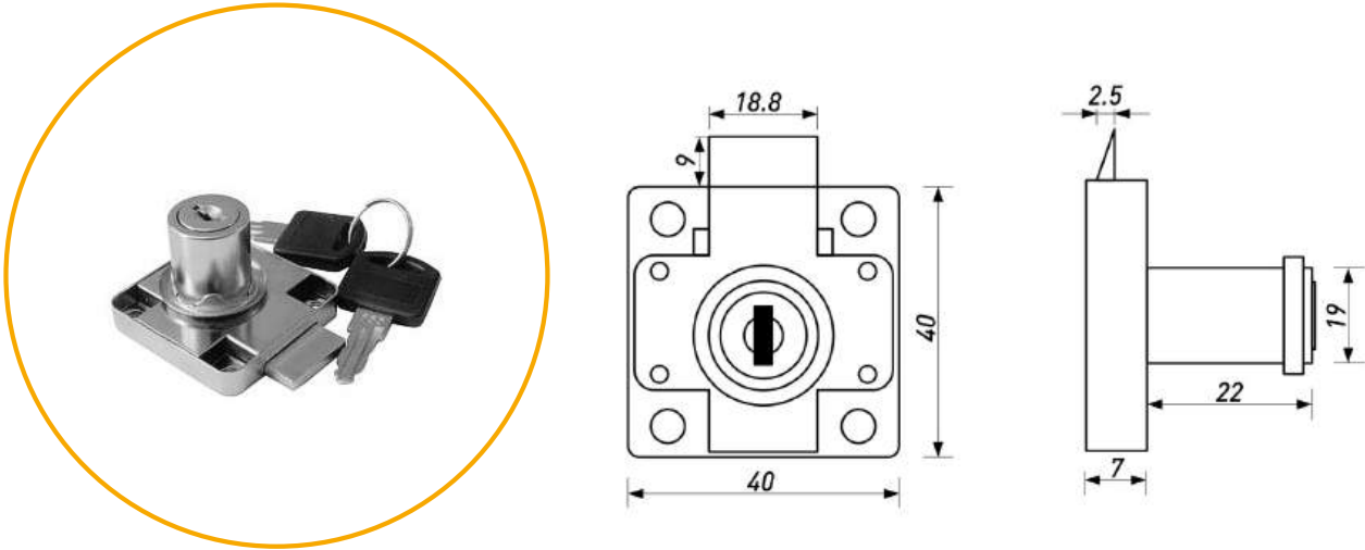
ЗАМОК МЕБЕЛЬНЫЙ № 138
