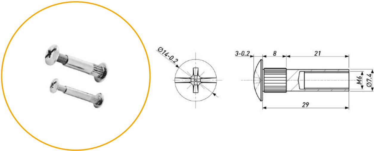
СТЯЖКА МЕЖСЕКЦИОННАЯ
