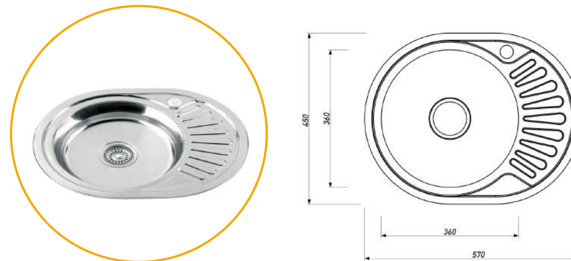
МОЙКА ОВАЛЬНАЯ (ЛЕВАЯ)
